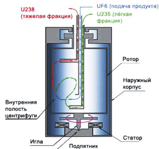
Схема работы центрифуги для производства урана-235.
